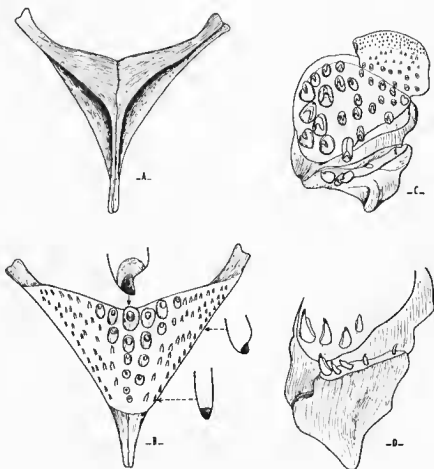
FIG. 18. — Ptychochromoides n. gen. beisleianus (Boulenger). A : Pharyngien inférieur, face interne et synarthrose. B : Pharyngien inférieur, face externe. C : Pharyngien supérieur, vue de dessus. D : Vue de 3/4 avant.
